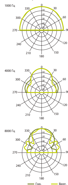
Гор./верт. диаграммы направленности
