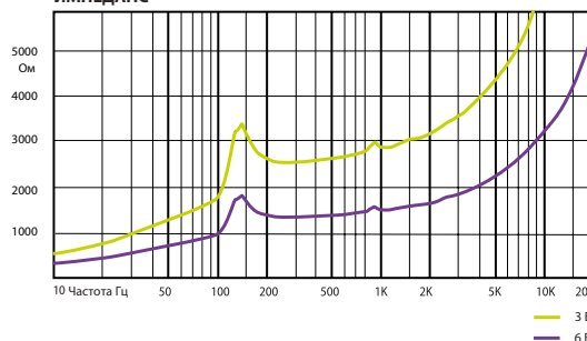
ИМПЕДАНС
