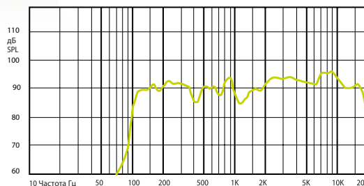
ЧАСТОТНАЯ ХАРАКТЕРИСТИКА
