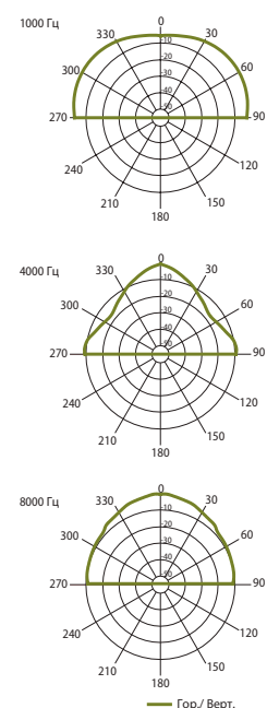
Гор./Верт. диаграммы направленности
