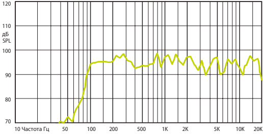
ЧАСТОТНАЯ ХАРАКТЕРИСТИКА
