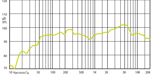
ЧАСТОТНАЯ ХАРАКТЕРИСТИКА
