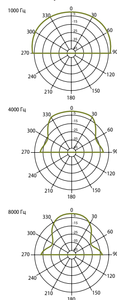
Гор./Верт. диаграммы направленности
